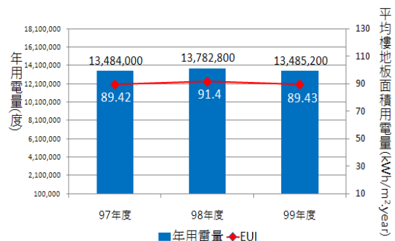
圖 6.7 校區總用電量與 EUI
