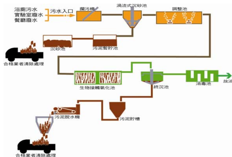
圖 4.2 污水處理流程
