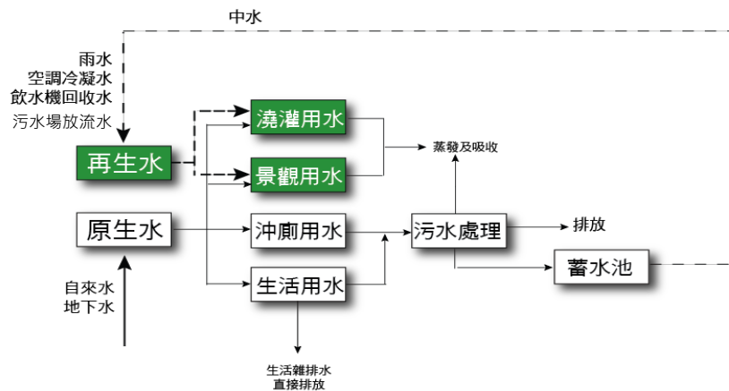
圖 6.13 用水平衡圖
