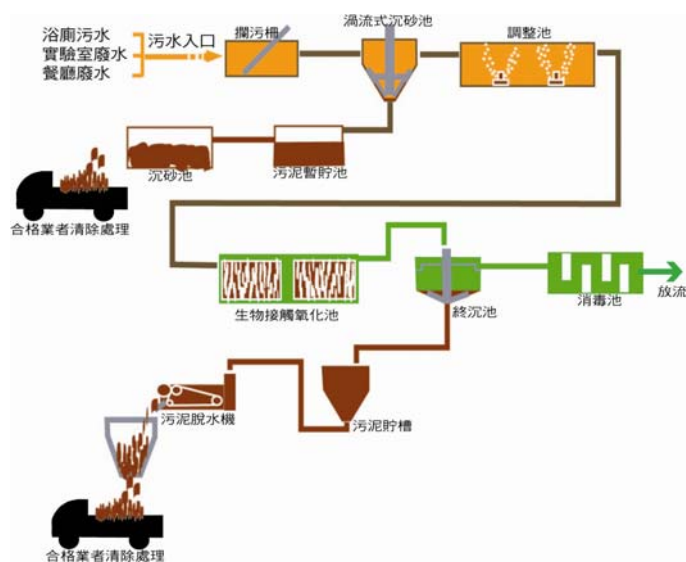
圖 4.2 污水處理流程
