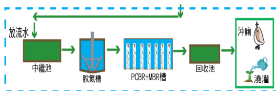
圖 6.14 中水回收設施處理流程
