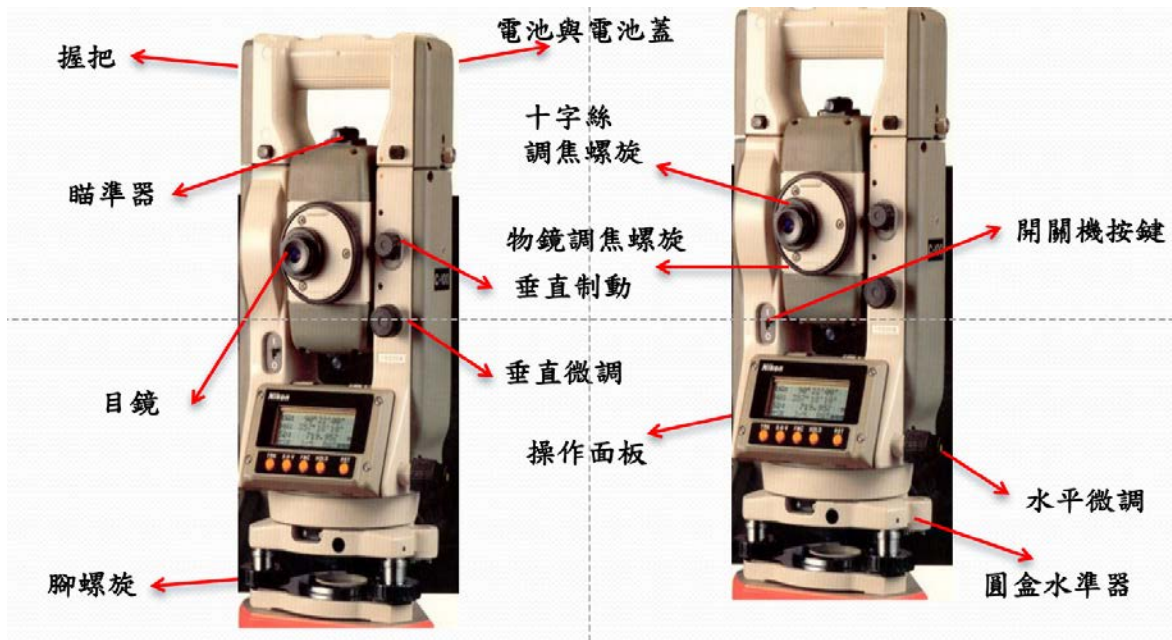
Nikon C-100 之儀器解說圖
